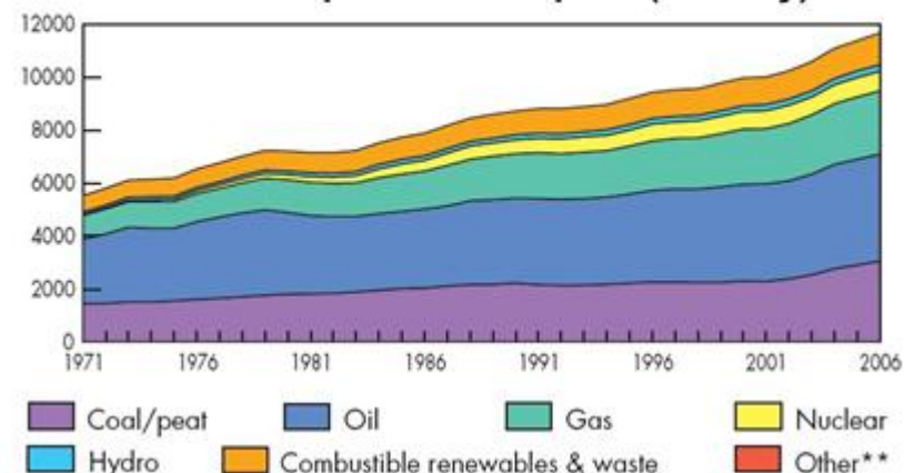
Динамика производства общемирового объема первичной энергии (по типу)
