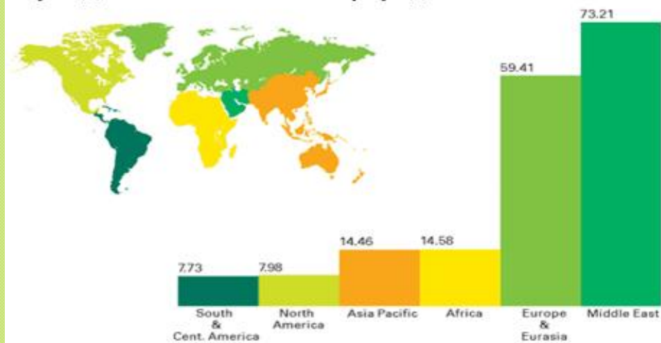
Карта доказанных запасов природного газа на 2008 г.
